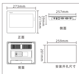
SK-102HE (V3.0)
