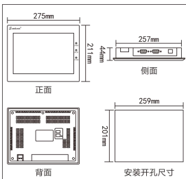
SK-102HS
