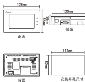
EA-043A
