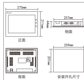
SK-102HG
