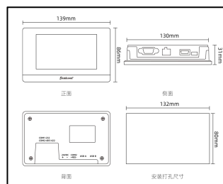
SK-043QE/QT
