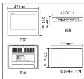
SK-102HS (V3.0)
